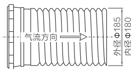
图(4)烟管示意图
