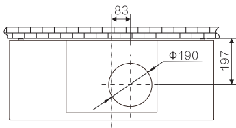
图(3) 橱柜及吊顶开孔俯视图
