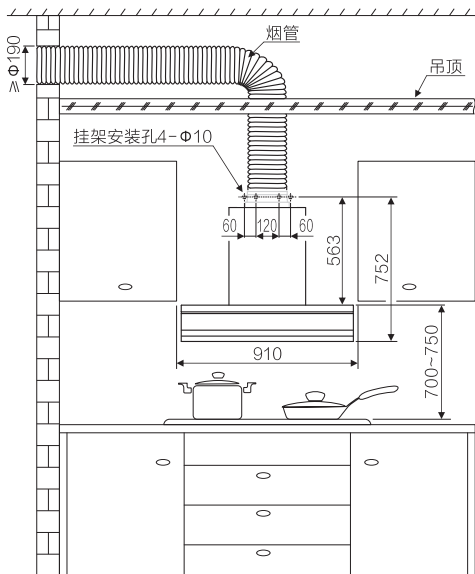
图(1) 橱柜安装正视图
