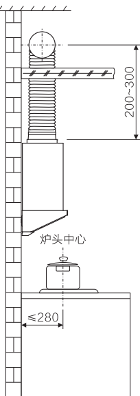
图(2) 橱柜安装侧视图
