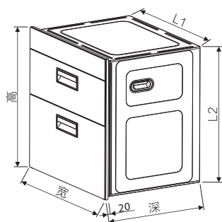
产品尺寸图
