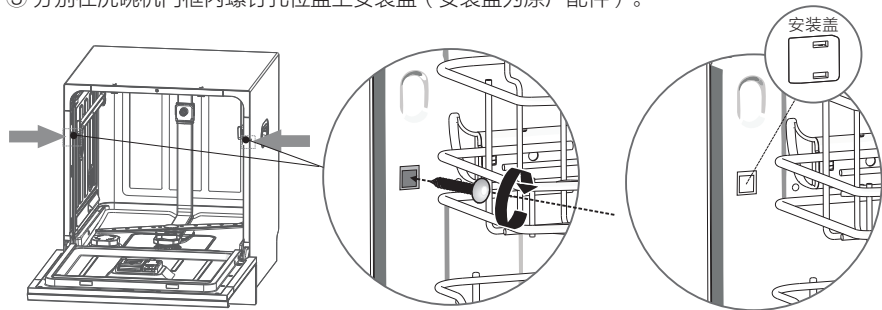
左右两边各一颗螺钉(4x25mm)
