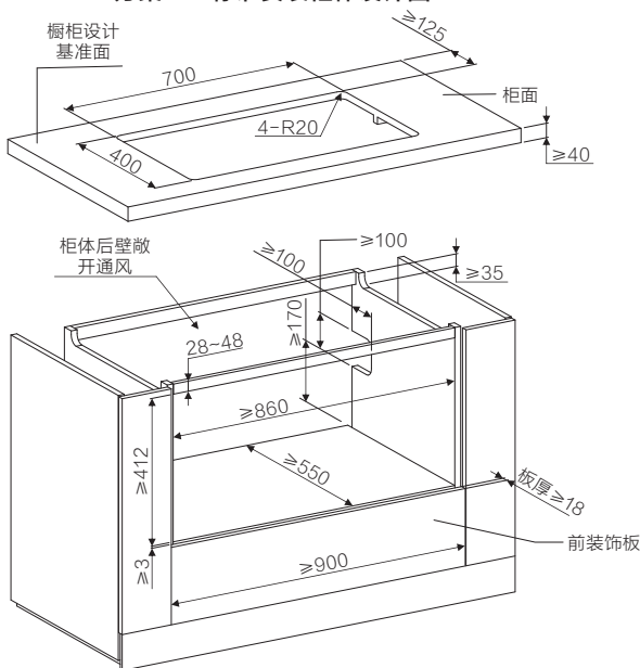
方案二：增加隔板安装柜体设计图
