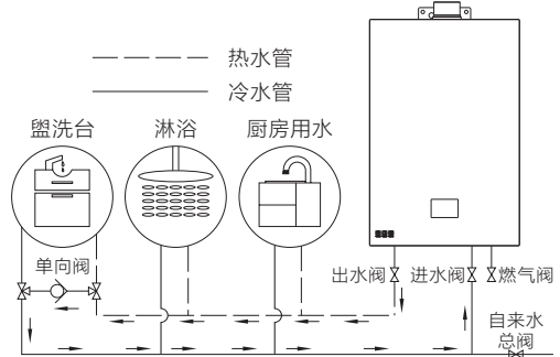
两管安装 图（1）
