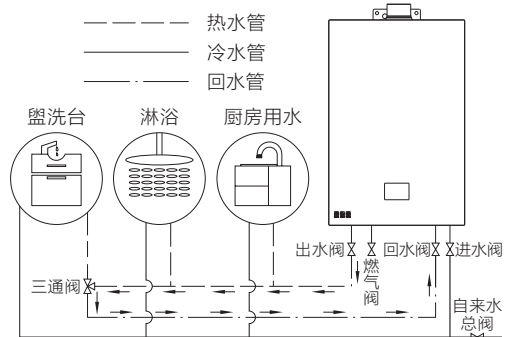
三管安装 图（2）
