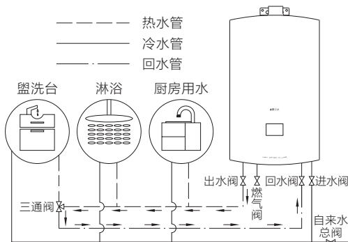
三管安装 图（2）
