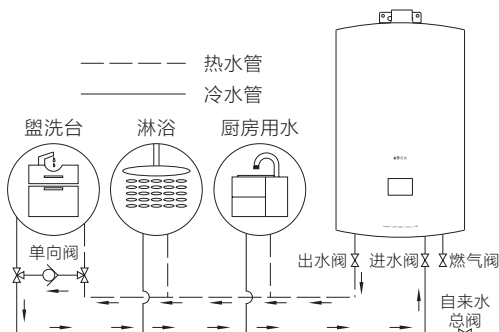
两管安装 图（1）
