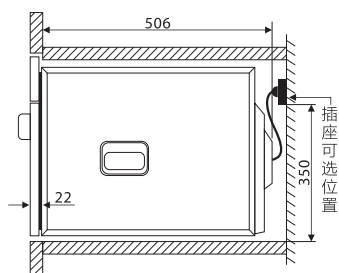
安装侧视图
