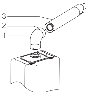
图3 给排气管管安装示意图
