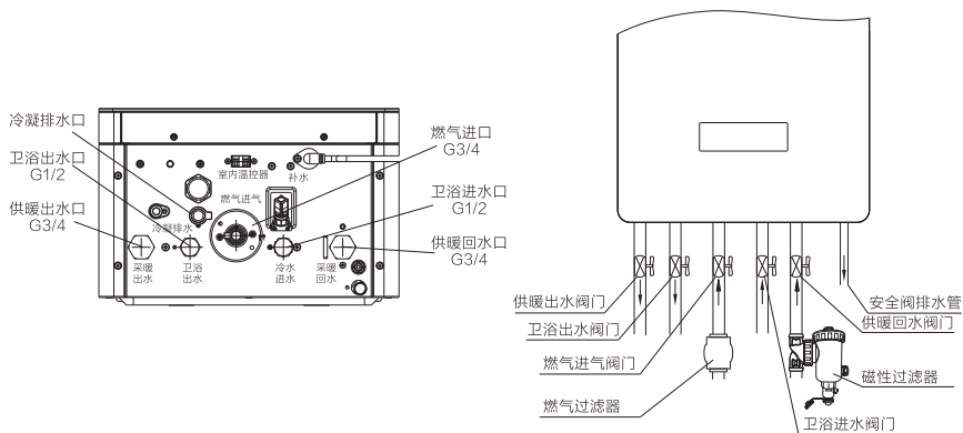
图1 管道示意
