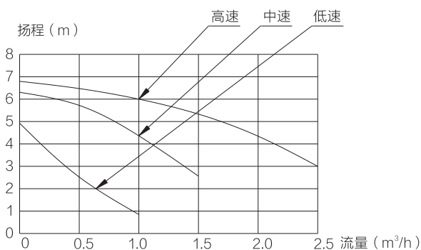
7m循环水泵特性曲线
