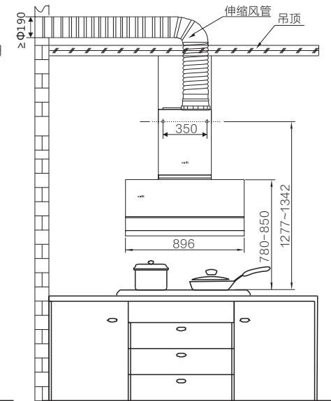
图（1b）平推安装图示（选配）
