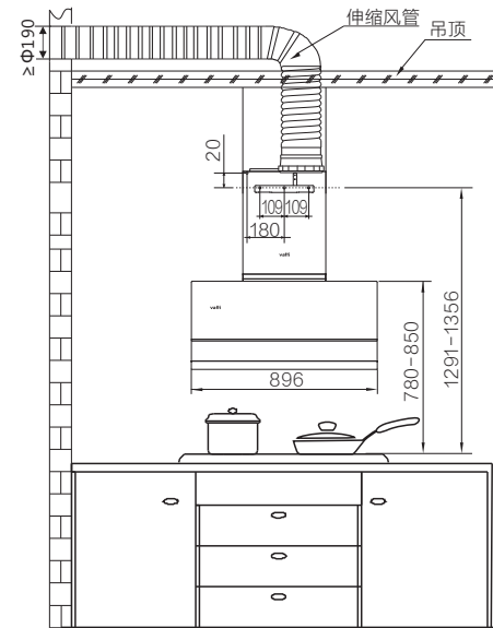
图（1a）挂架安装图示（标配）
